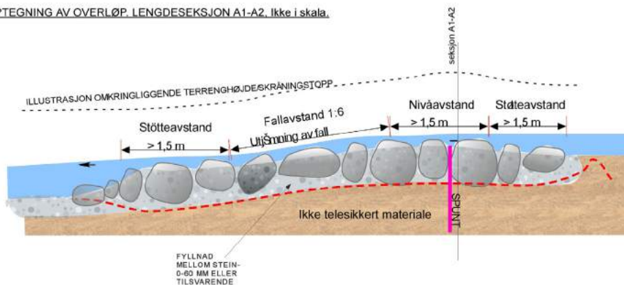
11 Våtmarkens utløp sett forfra og fra siden.
