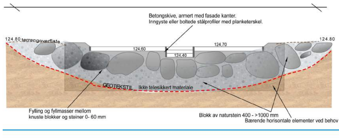
PRINSIPTEGNING AV OVERLØP. LENGDESEKSJON A1-A2. Ikke i skala.
