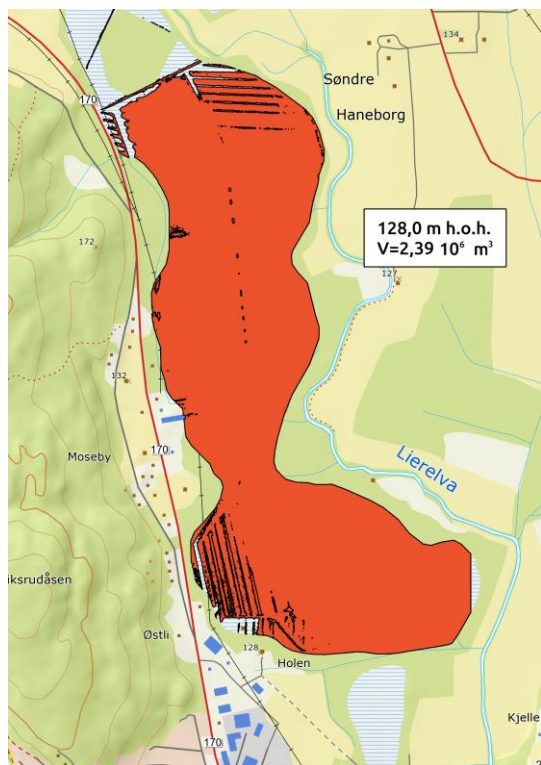
Figur 7: Areal som overflømmes ved begrenset utløp lagt på 128 moh. Fordrøyningsvolum ca 23900000m 3 .
