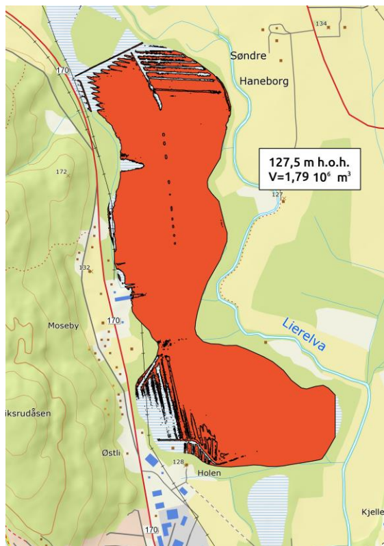
Figur 6: Areal som overflømmes ved begrenset utløp lagt på 127,5 moh. Fordrøyningsvolum ca 17900000m 3 .
